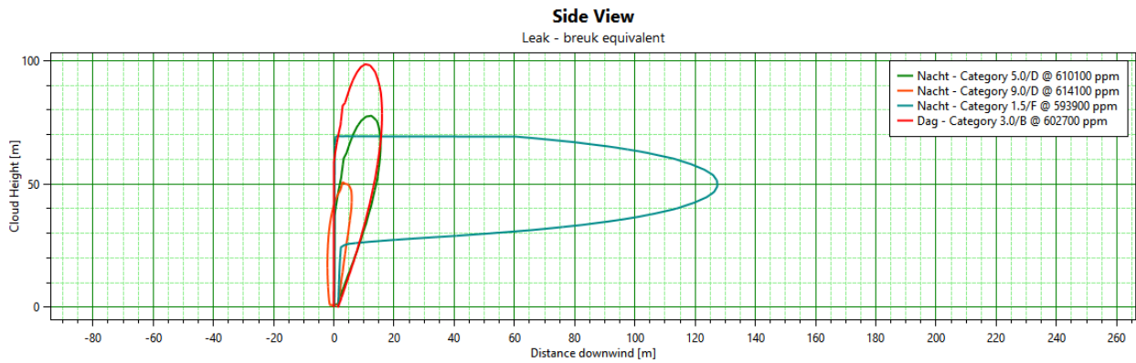
Figuur 7-11 Zijaanzicht verticale breuk
