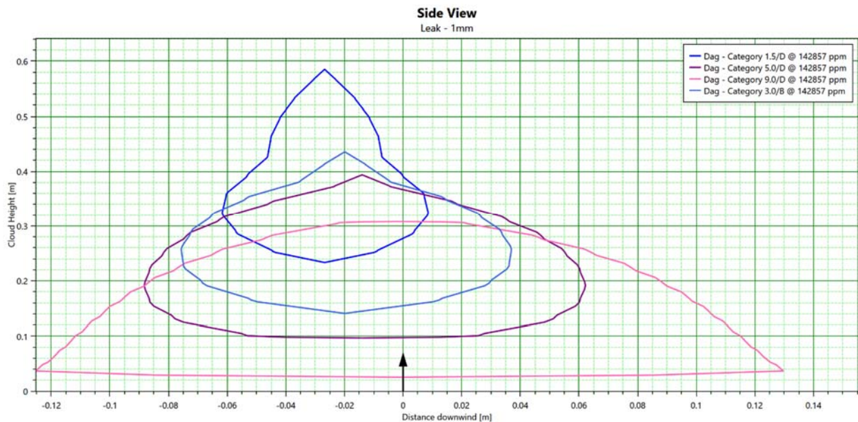
Figuur 7-1: 1mm lek – Dispersiecontouren bij dag
