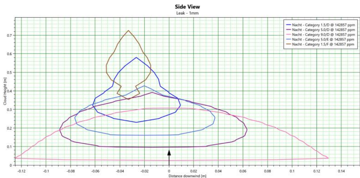
Figuur 7-2: 1mm lek – Dispersiecontouren bij nacht
