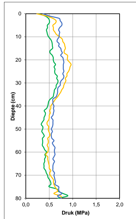
Figuur 5-7: Indringingsweerstand gemeten onder rijplatenbaan en presentatie alle gemiddelde waarden
